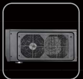
Überdruckdesign zur ausgezeichneten Kühlung, Geräuscharm und Verhinderung von Staubbildung
